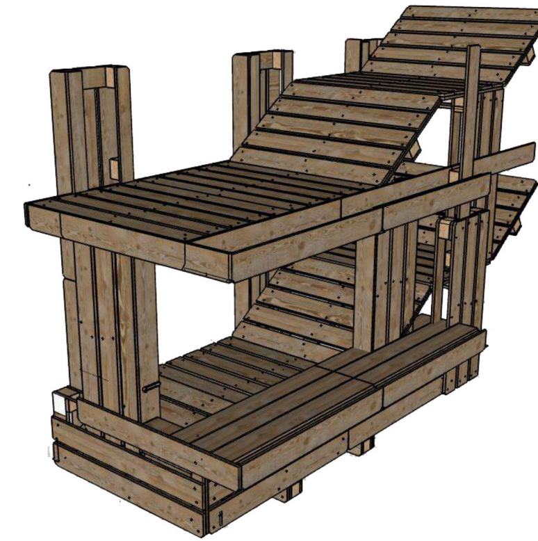
ASSISES LOUNGES PLATEAUX ÉPAIS INCORPORANT DES PERSIENNES
