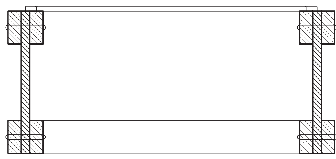
Détails 1:10
